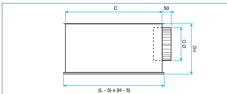
Diffuseur SF 785 avec plénum RE - Fixation F0 - montage en dalles de plafonds suspendus
