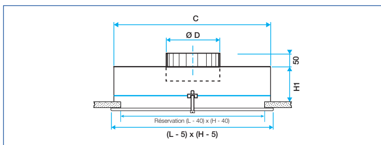
Diffuseur SF 785 avec plénum RT - fixation F7 - montage en BA13
